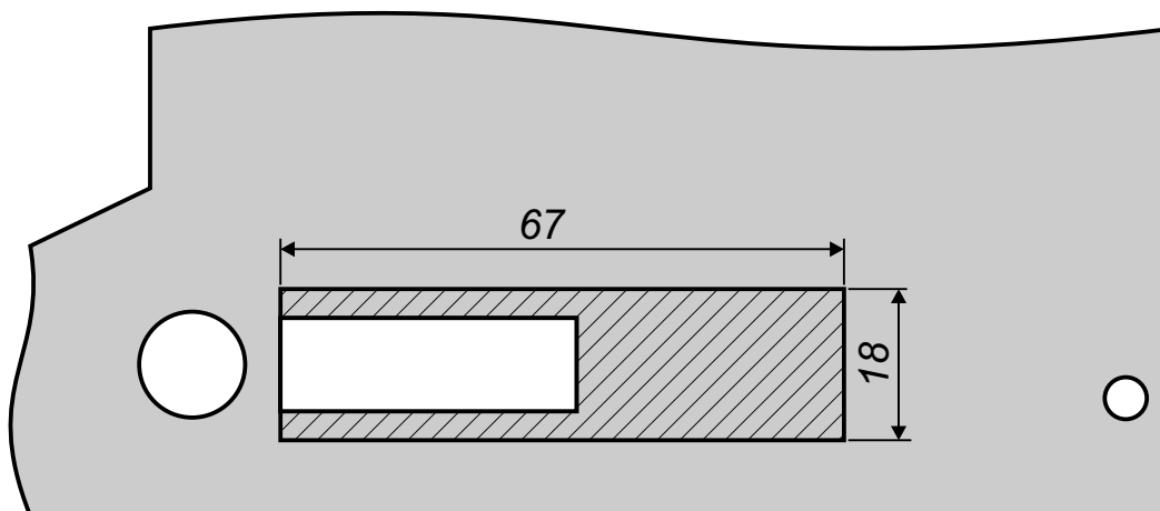
Рис. 6. Доработка передней панели магнитофона.
