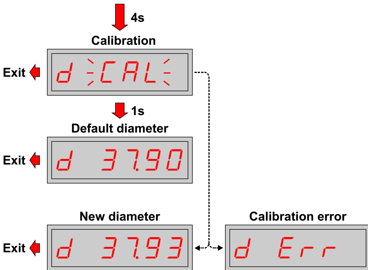
Рис. 4. Калибровка диаметра ролика.
