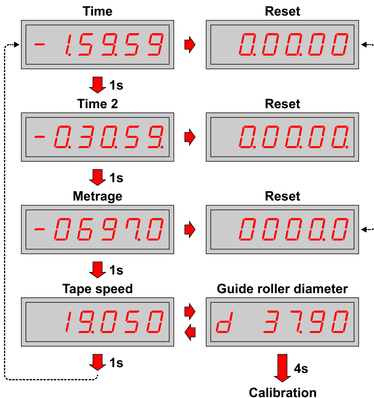
Рис. 3. Дополнительные режимы работы счетчика.
