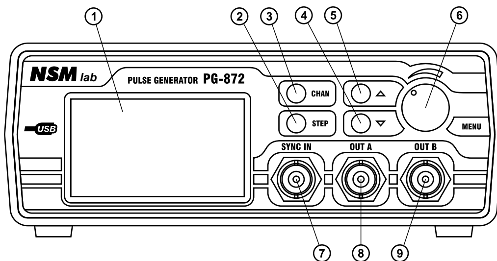
Рис. 1. Внешний вид передней панели генератора PG-872.
