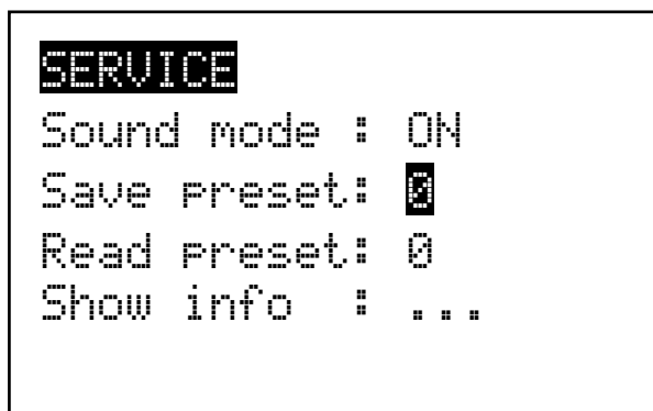
Рис. 9. Меню сервиса.
